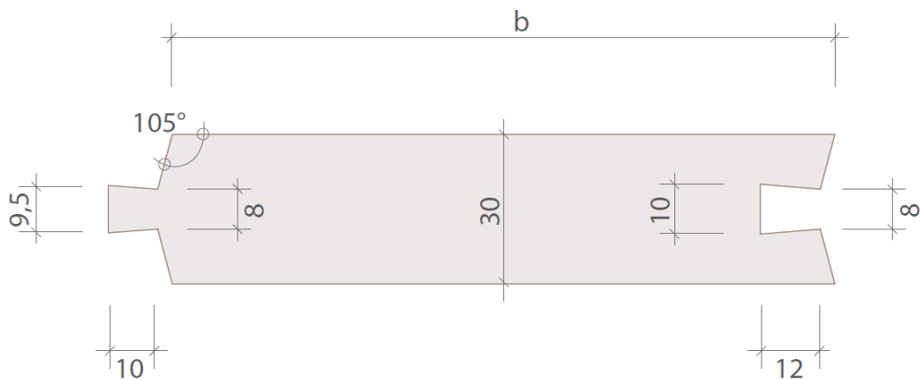
Einzelbrett des GFM-Systems mit Darstellung Nut/Feder
