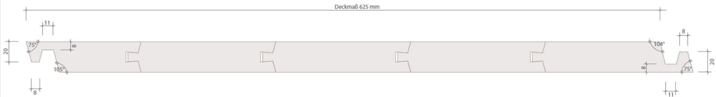
Plattenquerschnitt der GFM-Platten mit Darstellung des Einhängesystems
